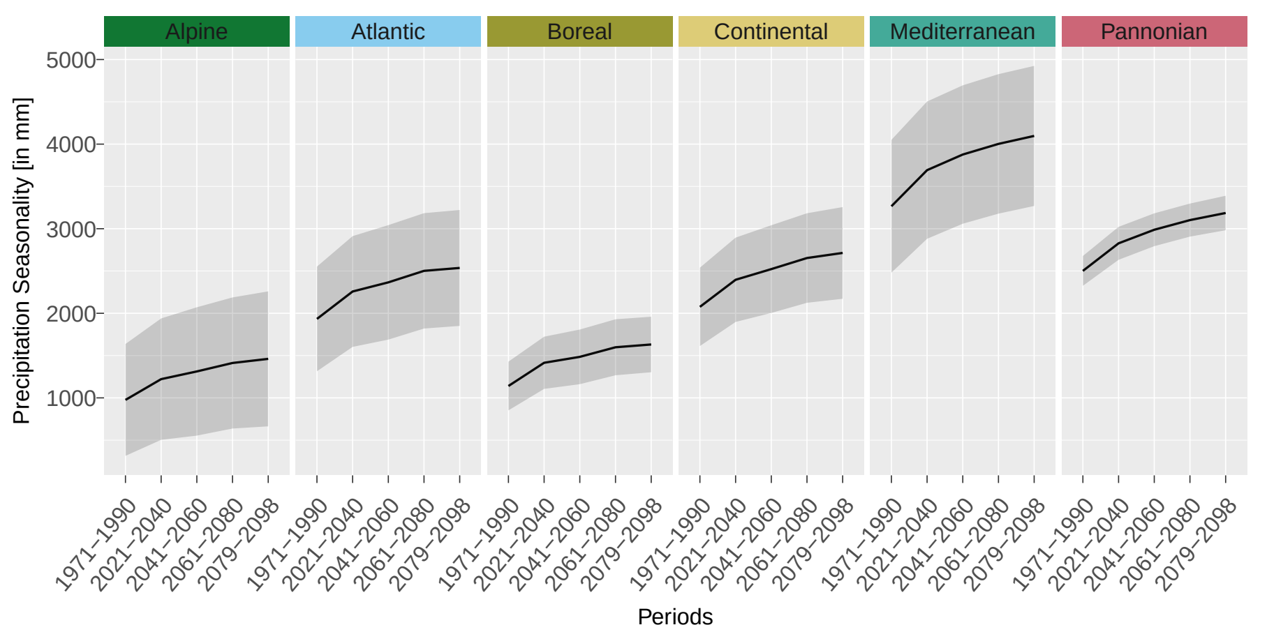
(d) Precipitation Seasonality
